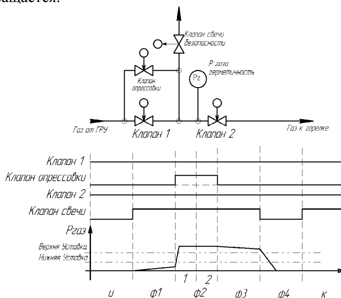
Рисунок 5 – Выполнение контроля герметичности по 2 уставкам (АМАКС)
