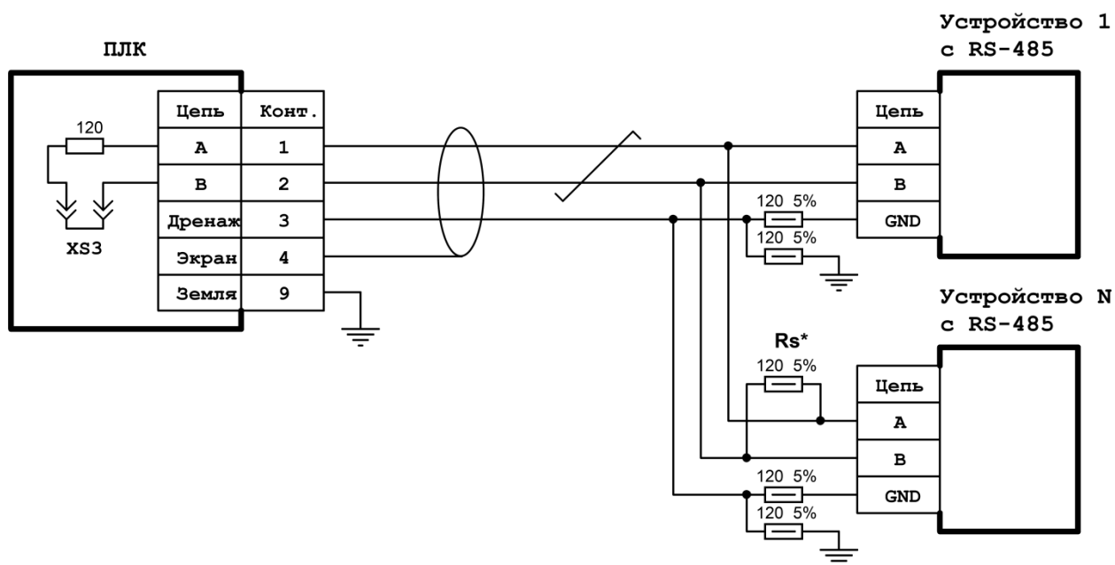
Рисунок П2-2. Схема подключения экранированной линии RS-485
