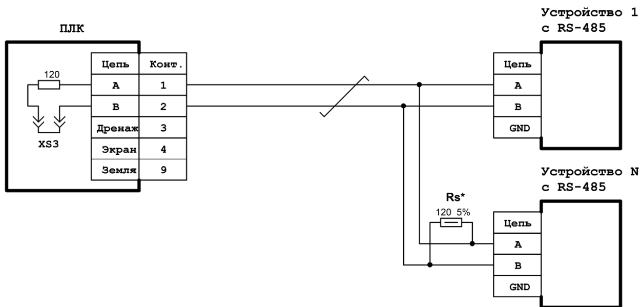
Рисунок П2-1. Простая схема подключения линии RS-485
